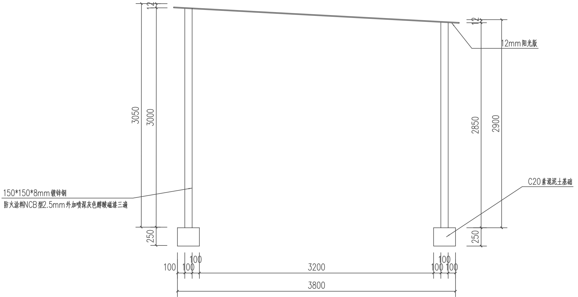
车棚侧立面
